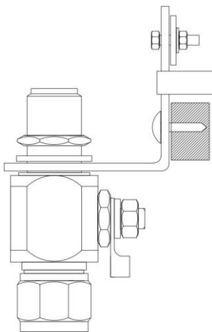
Рисунок 3.2 Крепление грозоразрядника
