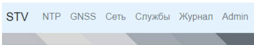
Рисунок 7 — Меню навигации.
