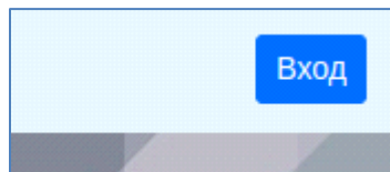
Рисунок 5 — Кнопка Вход.
