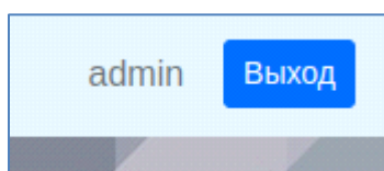
Рисунок 8 — Кнопка Выход.
